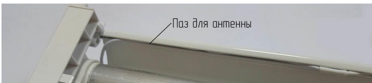
Рис. Установка трубы с мотором в изделие. (Показано без ткани и доп. профиля для наглядности)
