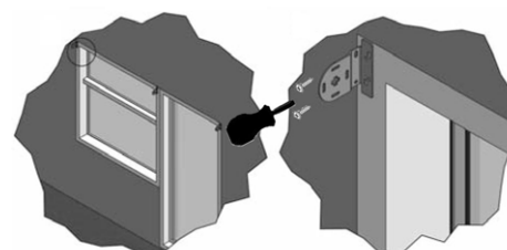
Рис. 7. Установка кронштейнов для DOUBLE AMG
